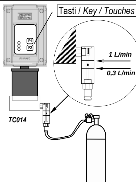
Fig. 3 - Tester di calibrazione / Calibration Tester / Kit de Calibration
