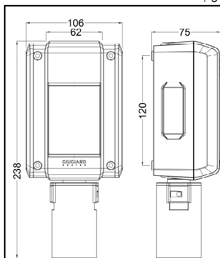
Fig. 1 - Dimensioni / Size / Dimensions
