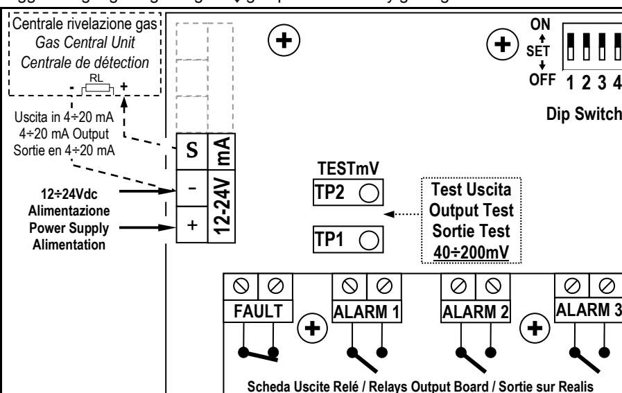
Fig. 2 - Schema di collegamento / Wiring diagram / Schéma
