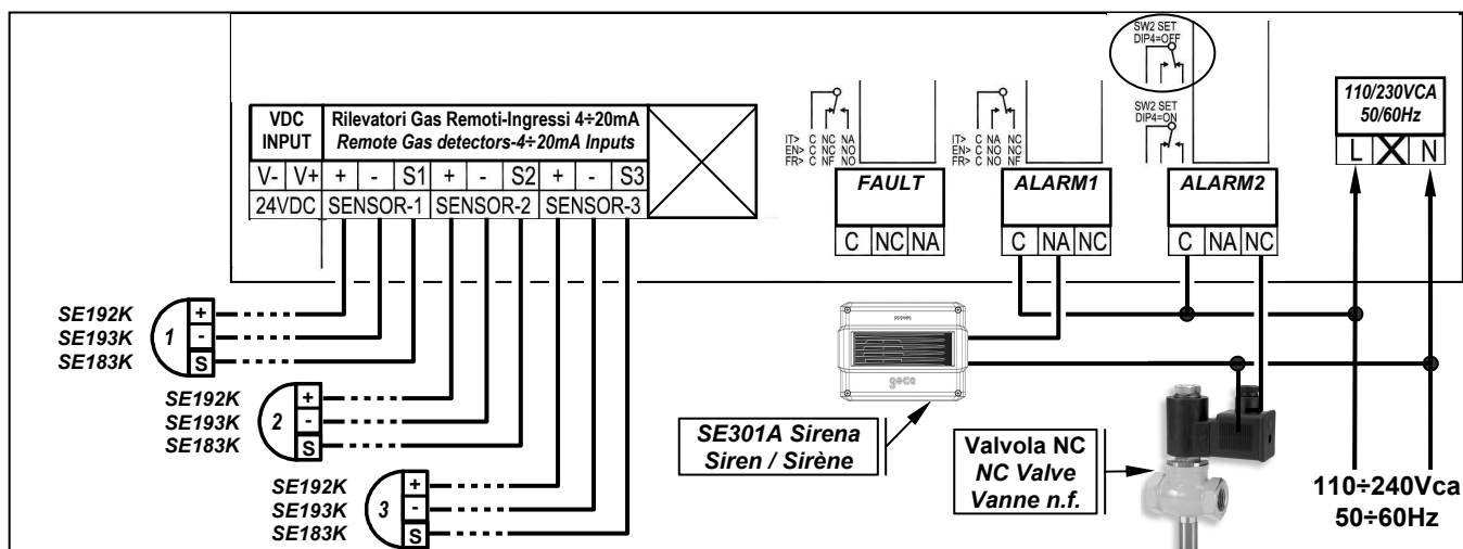
Fig. 5 - Collegamento con valvola a riarmo manuale Norm.Chiusa / Wiring diagram with a normally closed manual resetting valve / Schéma avec vanne à réarmement manuel norm.fermée
